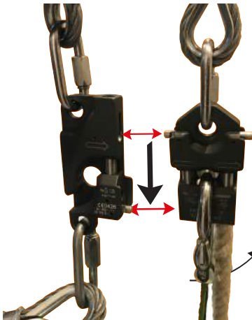
2 - DECONNEXION PARTIE MOBILE DISCONNECTION MOVING PART
